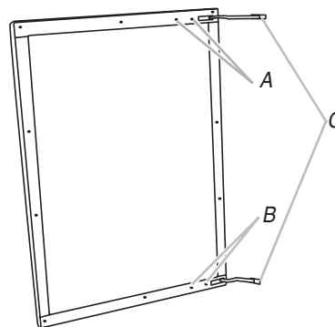
A. Vis de charnière supérieure (2) B. Vis de charnière inférieure (2) C. Charnières (2)
